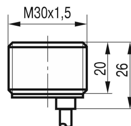
Габаритный чертеж
