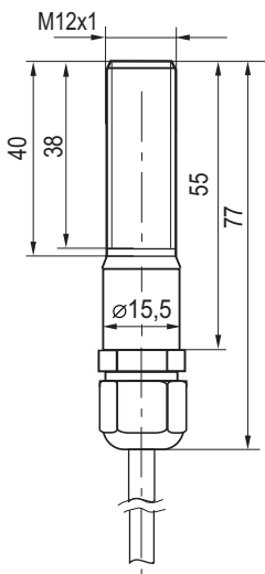
Габаритный чертёж
