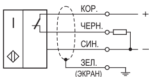
Схема подключения активной нагрузки
