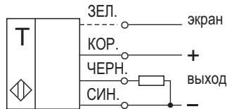
Схема подключения
