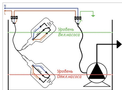
Откачивание из емкости FLRF-WOLXX3M-FCC-A
