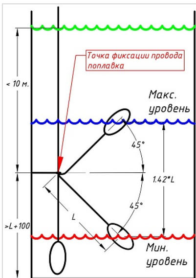
Монтаж и настройка FLRF-WOLXX3M-FCC-A
