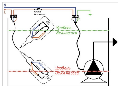
Защита насоса от сухого хода FLRF-WOLXX3M- FCC-A
