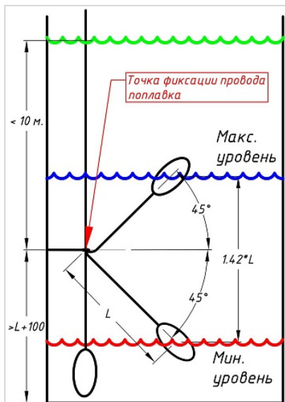
Монтаж и настройка FLRF-WOLXX8M-FCC-A
