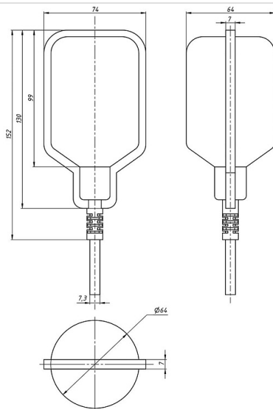
Размеры FLRF-WOLXX8M-FCC-A
