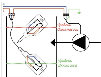
Заполнение емкости FLRF-WOLXX8M-FCC-A
