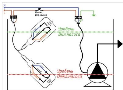
Защита насоса от сухого хода FLRF-WOLXX2M- FCC-A
