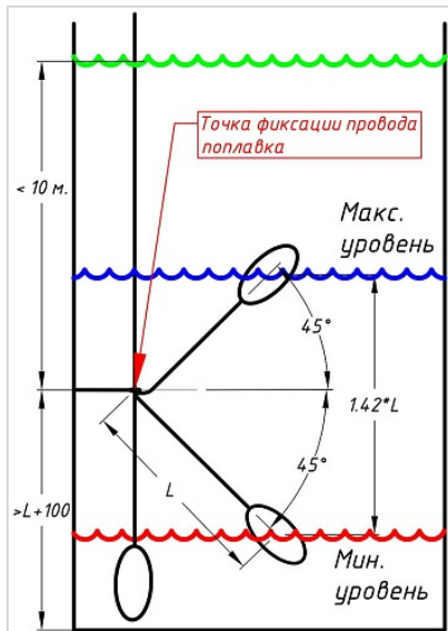
Монтаж и настройка FLRF-WOLXX2M-FCC-A
