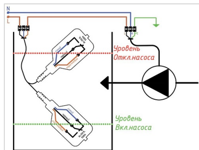
Заполнение емкости FLRF-WOLX15M-FCC-A
