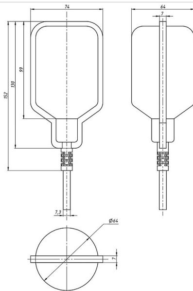
Размеры FLRF-WOLXX6M-FCC-A
