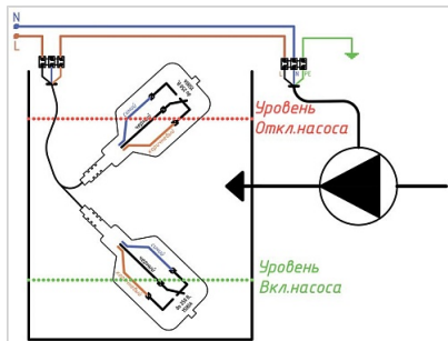
Заполнение емкости FLRF-XXXXX3M-FCC-A
