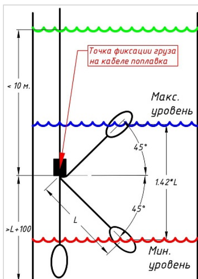
Монтаж и настройка FLRF-XXXXX3M-FCC-A
