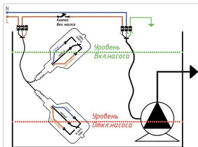
Защита насоса от сухого хода FLRF-XXXXX3M-FCC- A
