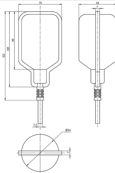
Размеры FLRF-XXXXX3M-FCC-A
