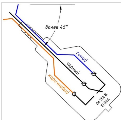
FLRF-WOLX20M-FCC-A, поплавок направлен вниз
