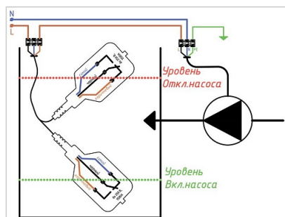
Заполнение емкости FLRF-WOLX20M-FCC-A
