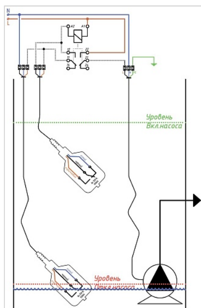
Насос выключен FLRF- WOLX20M-FCC-A
