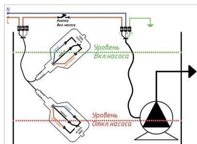
Защита насоса от сухого хода FLRF-WOLX20M-FCC- A
