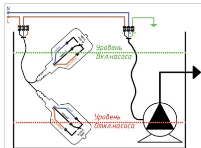
Откачивание из емкости FLRF-WOLX20M-FCC-A
