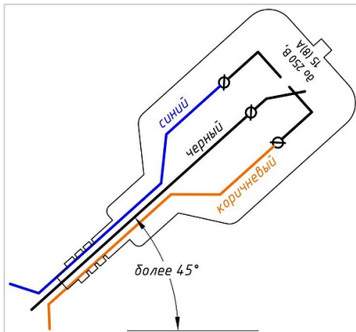
FLRF-WOLX20M-FCC-A, поплавок направлен вверх на угол более 45 град
