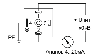
Схема соединений:
