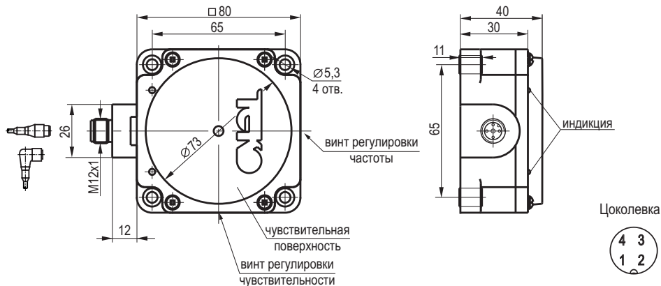
Габаритный чертёж
