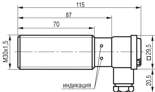
Габаритный чертеж
