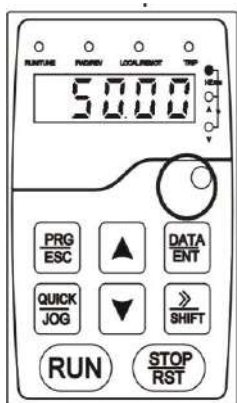
Stop state parameter display
