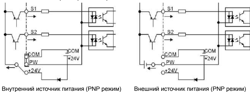
Рис. 4-18 PNP режим
