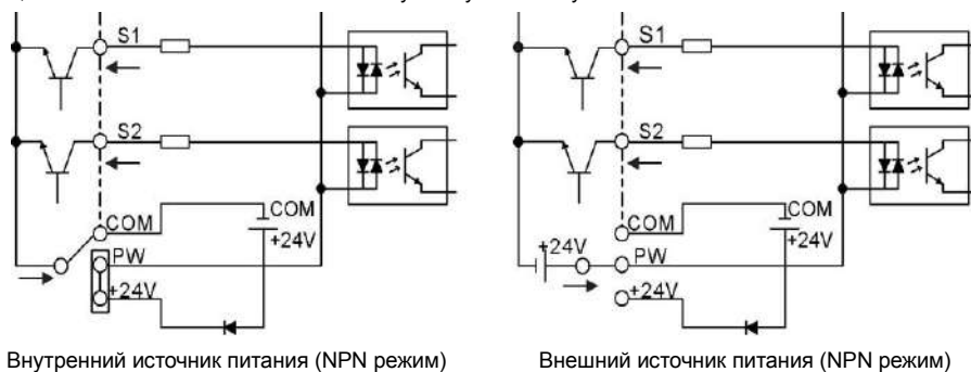
Рис. 4-17 NPN режимы
