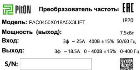
Рис. 3-4 Табличка ПЧ
