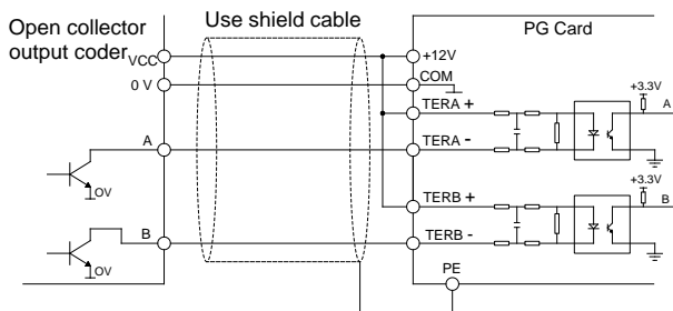
Рис. А-7 Схема подключения энкодера с открытым коллектором (3) Схема подключения энкодера с двухтактным выходом
