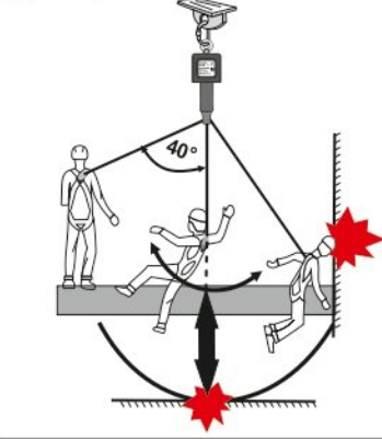
Рис. 7. Ограничения по использованию средств защиты втягивающего типа «АЛЬФА»
