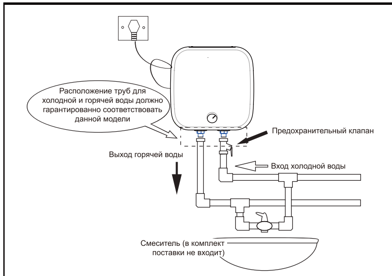
Монтажная схема для моделей, как серии SQ1, у которых горячая вода поступает вниз.
