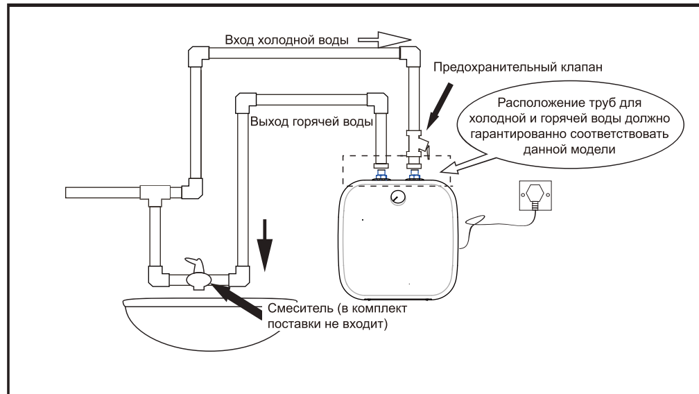
Монтажная схема для моделей, как серии SQ2, у которых горячая вода поступает навехр.
