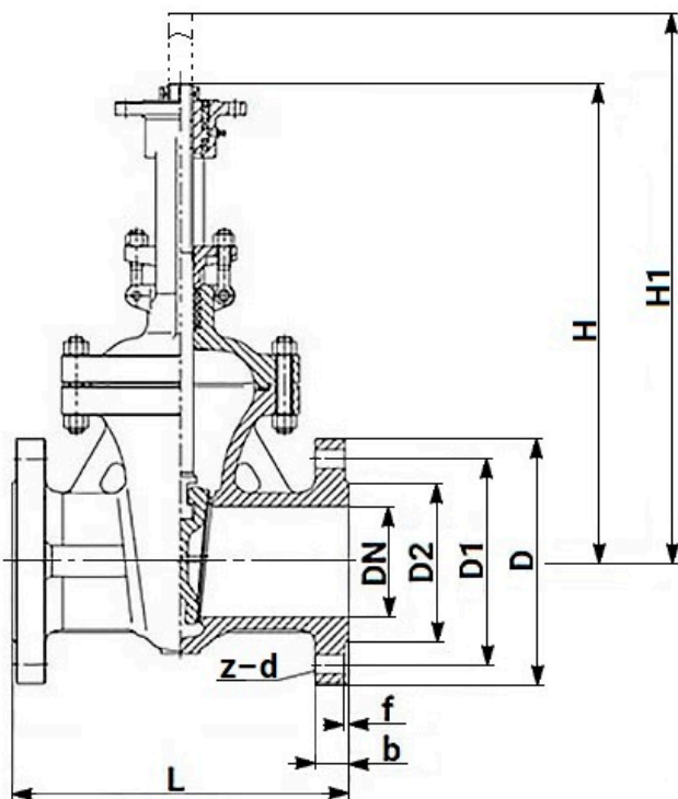
Рисунок 3 - Размеры изделия
