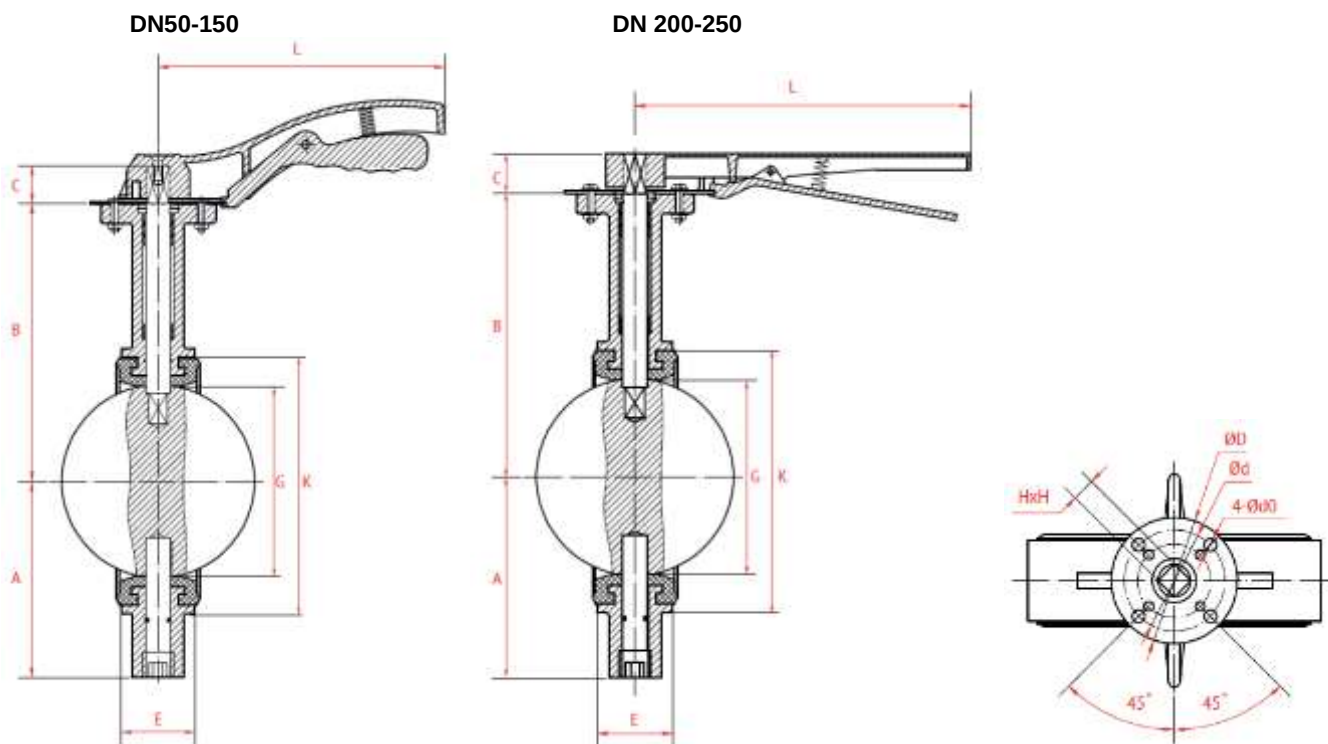
Основные параметры затворов с рукояткой DN50-250
