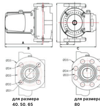
Рисунок 1 – Габаритные размеры
