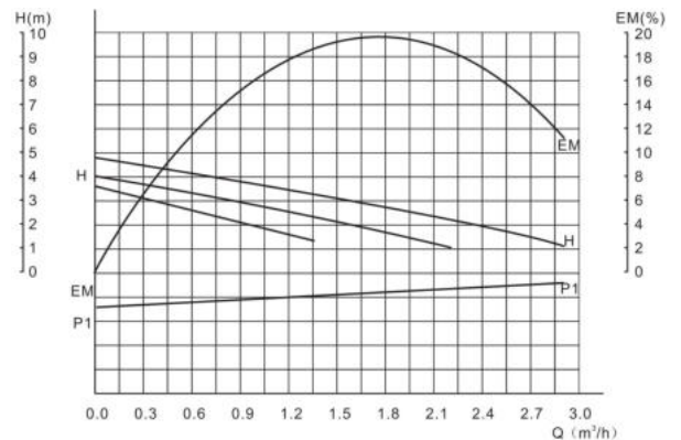
Рисунок 4 – График рабочих характеристик для моделей 25/4G-130, 25/6G-180
