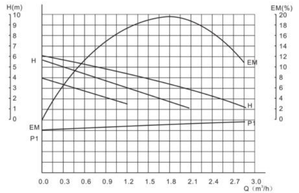
Рисунок 3 – График рабочих характеристик для модели 15/6G-130
