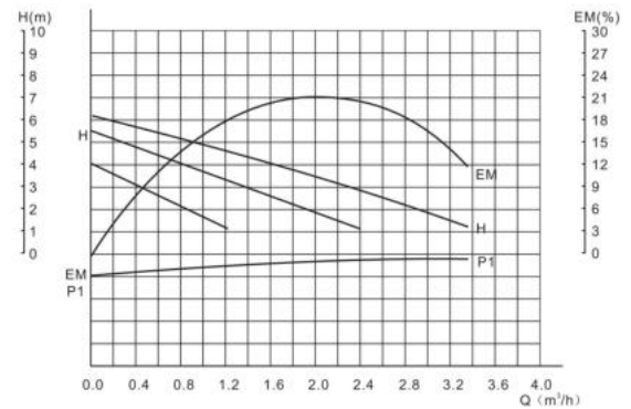
Рисунок 7 – График рабочих характеристик для модели 32/6G-180
