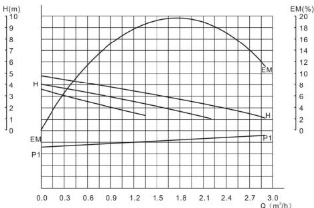
Рисунок 6 – График рабочих характеристик для модели 32/4G-180
