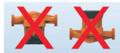
Рисунок 5 – Неправильная установка
