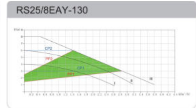
Рисунок 10А – График рабочих характеристик для модели RS 25/8EAY-130
