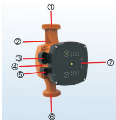
Рисунок 2 – Конструкция электронасоса
