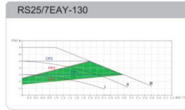
Рисунок 9А – График рабочих характеристик для модели RS 25/7EAY-130
