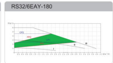
Рисунок 12А – График рабочих характеристик для модели RS 32/6EAY-180
