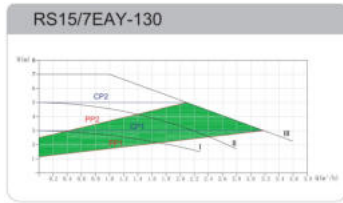
Рисунок 4А – График рабочих характеристик для модели RS 15/7EAY-130
