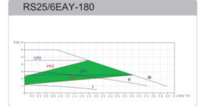
Рисунок 8А – График рабочих характеристик для модели RS 25/6EAY-180
