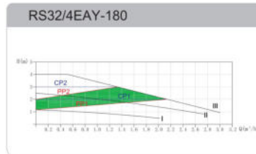
Рисунок 11А – График рабочих характеристик для модели RS 32/4EAY-180
