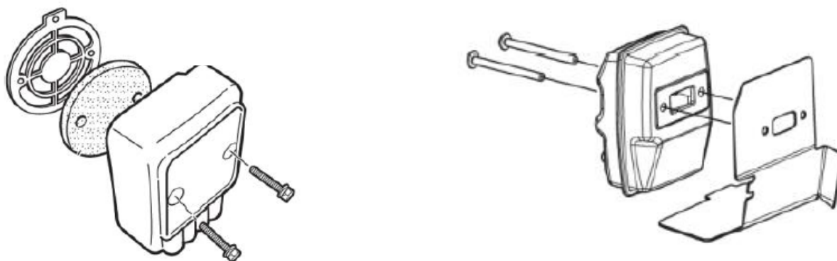
Рис. 24. Очистка фильтра
