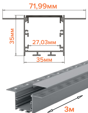
WAP-I-72/35/3000-A
