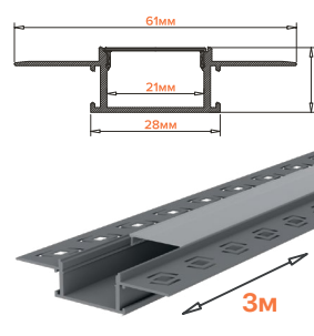
WAP-I-61/14/3000-A
