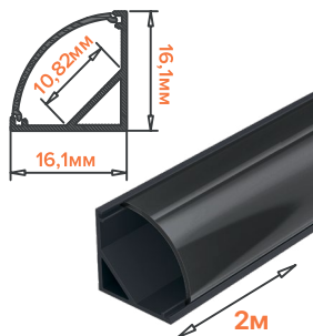
WAP-S-16/16/2000-B
