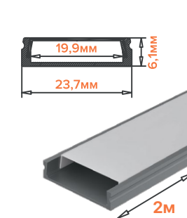
WAP-S-24/6/2000-A
