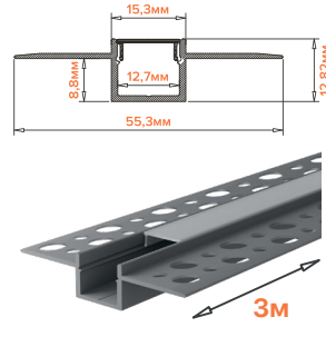
WAP-I-55/13/3000-A
