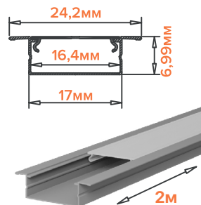
WAP-I-24/7/2000-A-LITE
