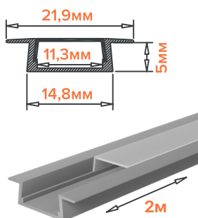
WAP-I-22/6/2000-A
