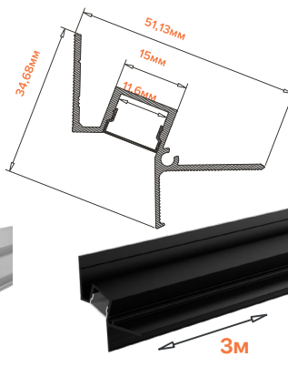
WAP-I-51/35/3000-B
