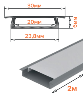
WAP-I-30/6/2000-A
