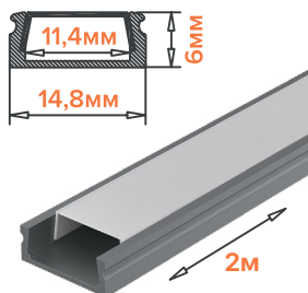
WAP-S-16/6/2000-A
