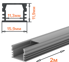
WAP-S-16/12/2000-A
