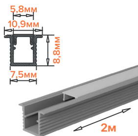
WAP-S-11/9/2000-A
