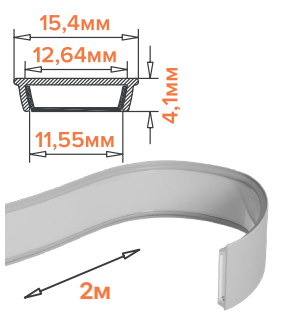
WAP-S-15/4/2000-A
