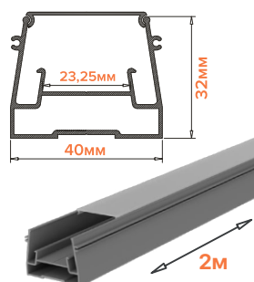
WAP-S-40/32/2000-A
