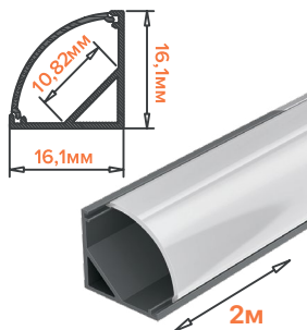
WAP-S-16/16/2000-A
