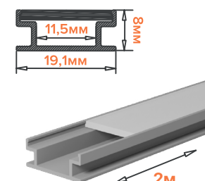
WAP-I/F-19/8/2000-A
