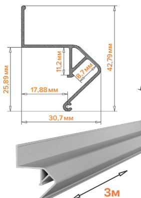
WAP-I-30/43/3000-A
