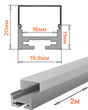
WAP-S/H-20/20/2000-A
