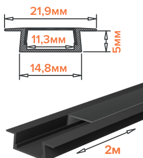
WAP-I-22/6/2000-B
