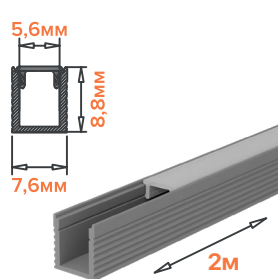
WAP-S-8/9/2000-A
