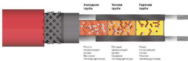
Рисунок 2.2 – Зависимость работы саморегулирующегося нагревательного кабеля REXANT от температуры
