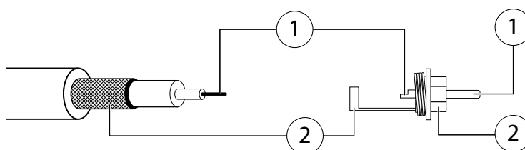
Рисунок 8.2 Схема расписки аудио кабеля и штекера RCA: 1 – Аудиосигнал; 2 – Экран/Земля
