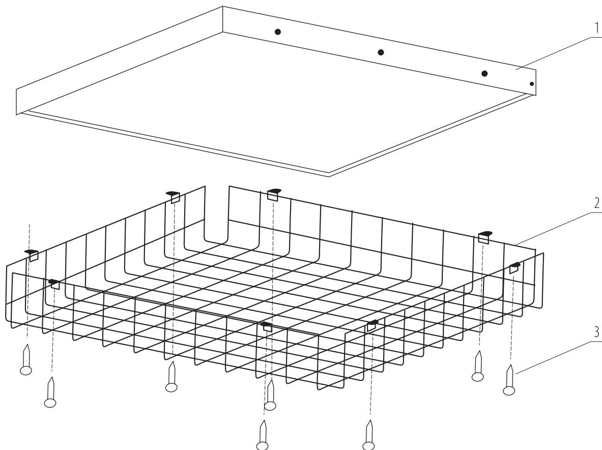
Рисунок 1. Схема монтажа защитной решётки
