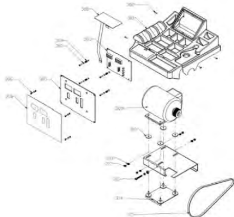
Двигатель/Верхняя крышка
