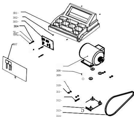
Двигатель/Верхняя крышка
