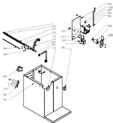
Платформа
