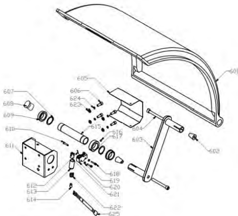
Защитный кожух
