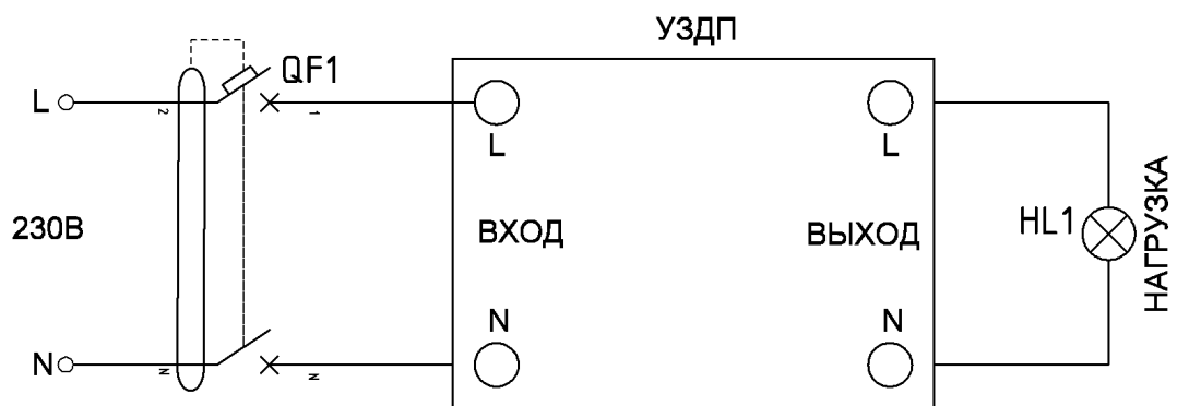
Рисунок Б.2 – Схема подключения УЗДП AFD9315 с дифференциальным автоматом (ДА)
