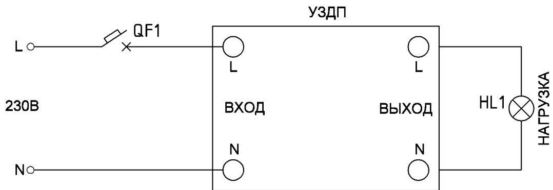
Рисунок Б.1 – Схема подключения УЗДП AFD9315 с автоматическим выключателем (АВ)
