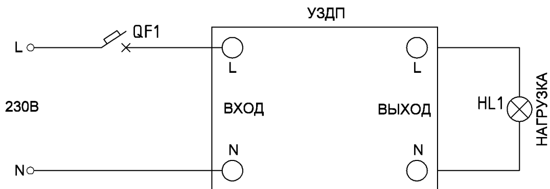
Рисунок Б.1 – Схема подключения УЗДП AFD9314 с автоматическим выключателем (АВ)
