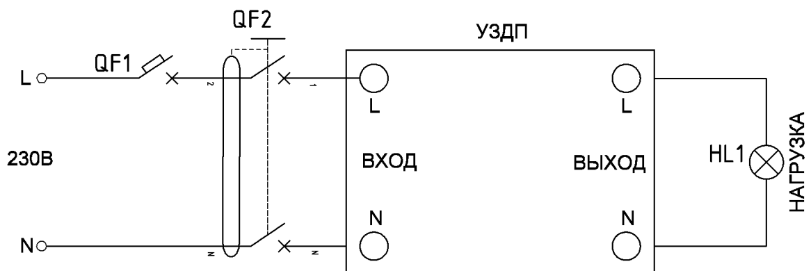
Рисунок Б.3 – Схема подключения УЗДП AFD9314 с устройством защитного отключения (УЗО)
