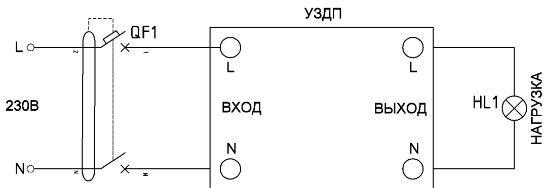
Рисунок Б.2 – Схема подключения УЗДП AFD9314 с дифференциальным автоматом (ДА)
