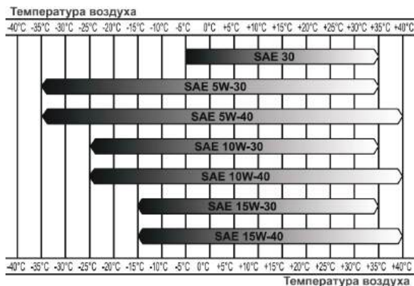
Рис. 5. Выбор масла
