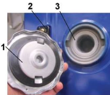
Рис. 3. Топливный бак 1- крышка топливного бака 2- указатель уровня топлива 3- фильтр
