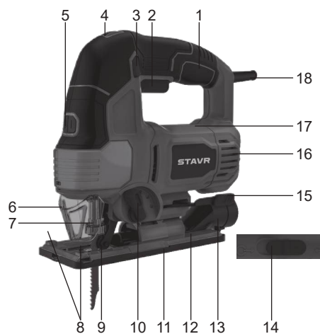
SJS 100-950LK
