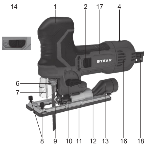
SJS 90-850K
