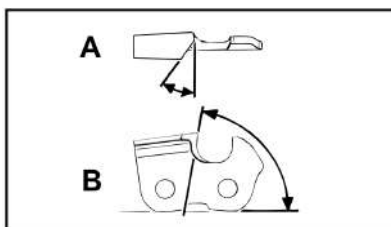
A —Угол заточки
