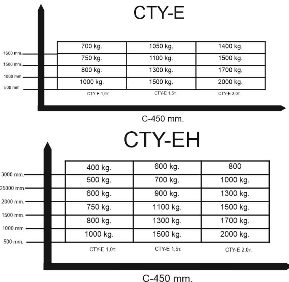
Рис. 2 – Кривые грузоподъемности
