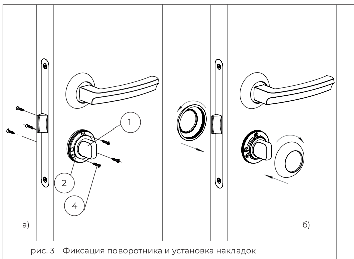
рис. 3 – Фиксация поворотника и установка накладок
