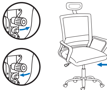
Регулировка жесткости качания / Swing stiffness adjustment / Тербелістің қаттылығын реттеу
