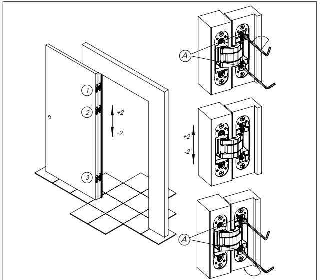
Рис. 3 — Вертикальная регулировка
