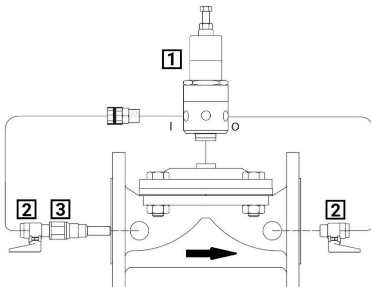
Рисунок 3 – Схема обвязки
