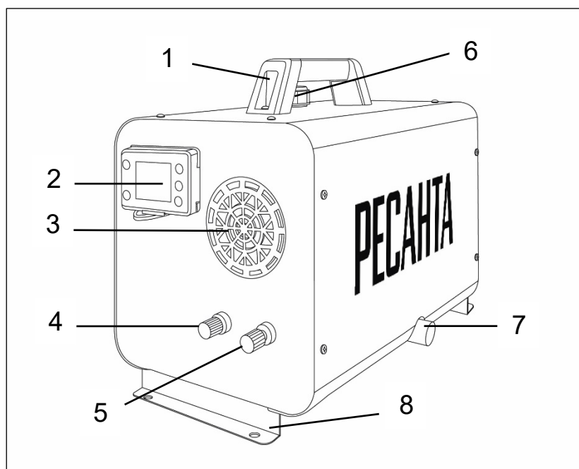
Рис. 1. Общий вид ТДПН.
