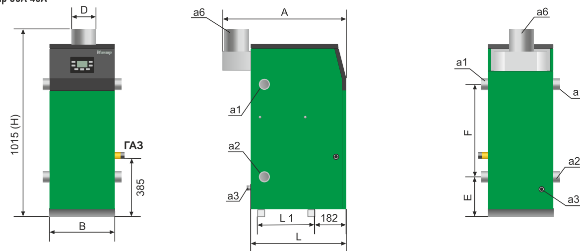
Размеры для Изнаир 50А 63А 80А 100А
