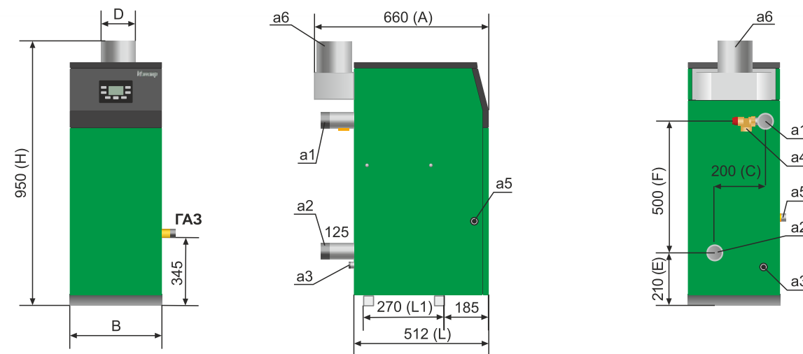
Размеры для Изнаир 30А 40А
