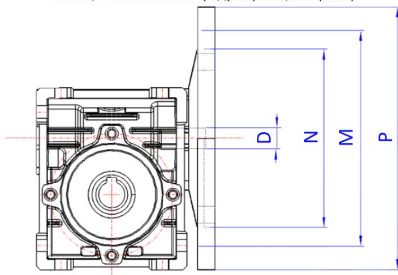
Фланцевое исполнение редуктора B5/B14 (РАМ)
