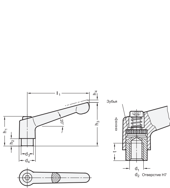
GN 300-с внутренней резьбой / с развернутым отверстием
