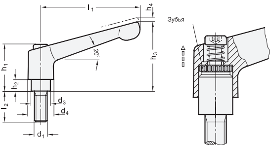
GN 300-с наружной резьбой
