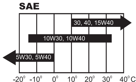
Рисунок 3.1 — Схема выбора марки масла в зависимости от температуры окружающего воздуха
