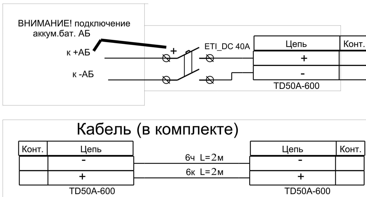
Рисунок 1.2 – Батарейный стеллаж Штиль BS-01. Схема электрическая соединительная
