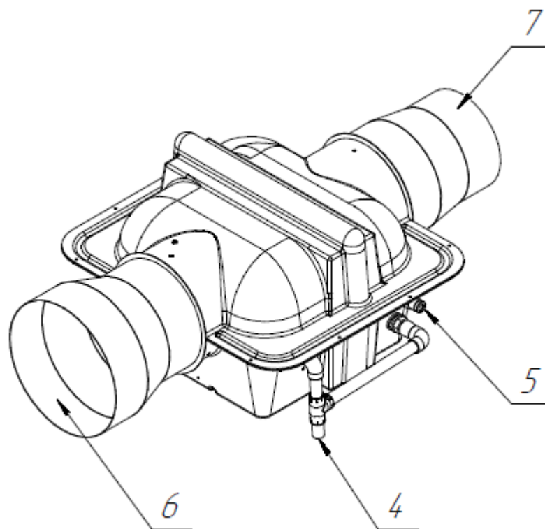
Рисунок 2.2. Модуль увлажнения ПК-6.ЭД
