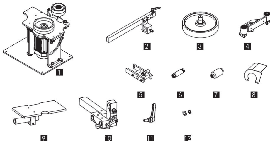
Рисунок 3. Комплектация станка.
