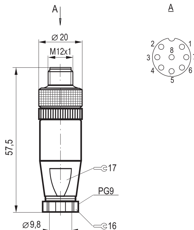
Габаритный чертеж
