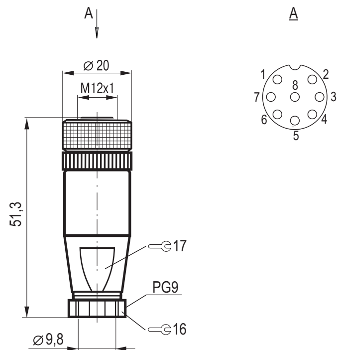
Габаритный чертеж
