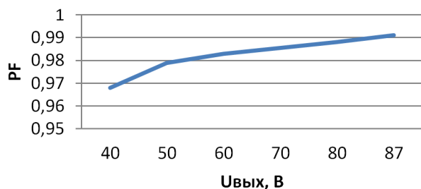
Зависимость коэффициента мощности от выходного напряжения
