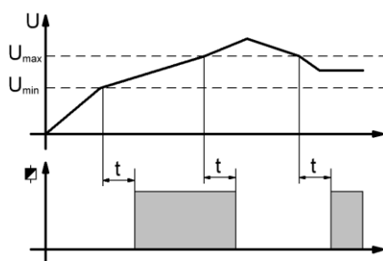
Рисунок 3 – Диаграмма работы реле контроля напряжения VCR22
