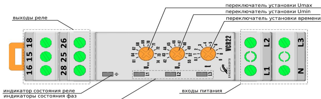
Рисунок 2 – Панель управления и индикации реле контроля напряжения VCR22
