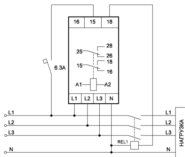
Рисунок 1 – Принципиальная схема подключения реле контроля напряжения VCR22
